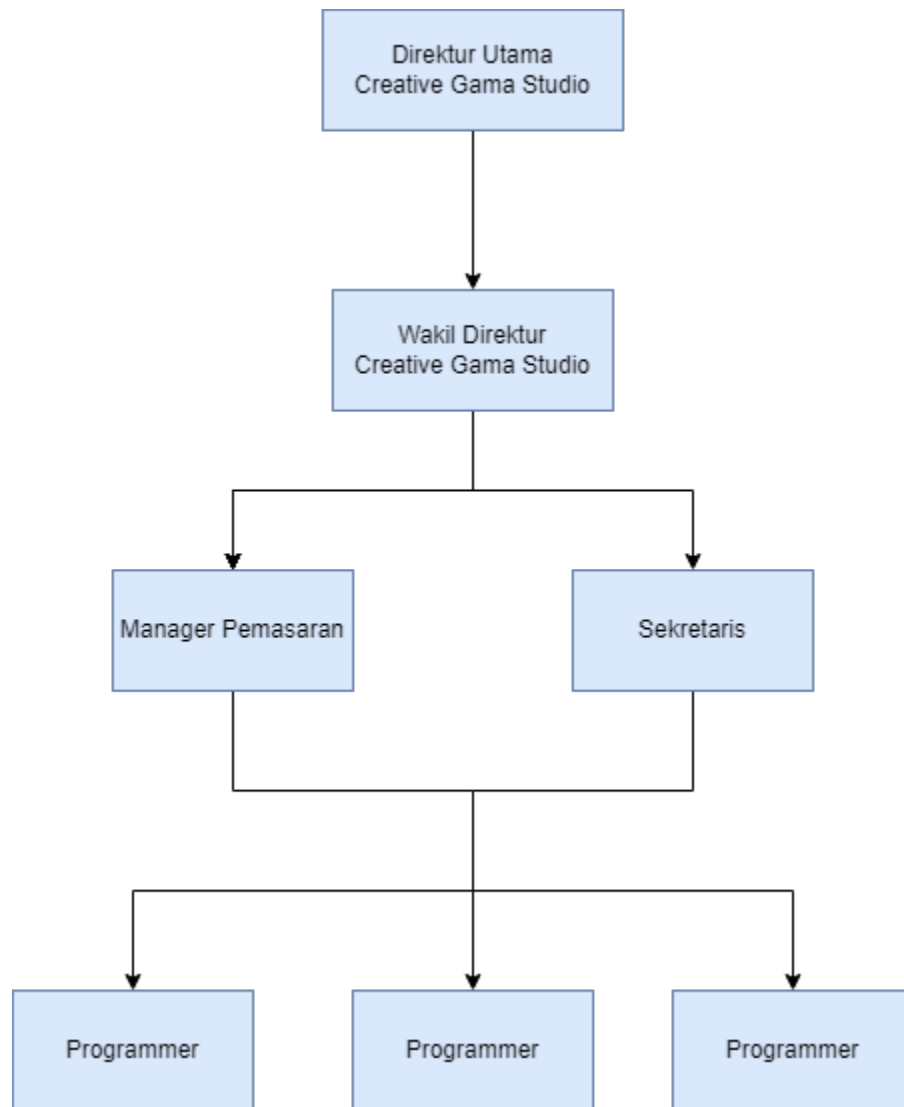
Gambar 2 Struktur Perusahaan
